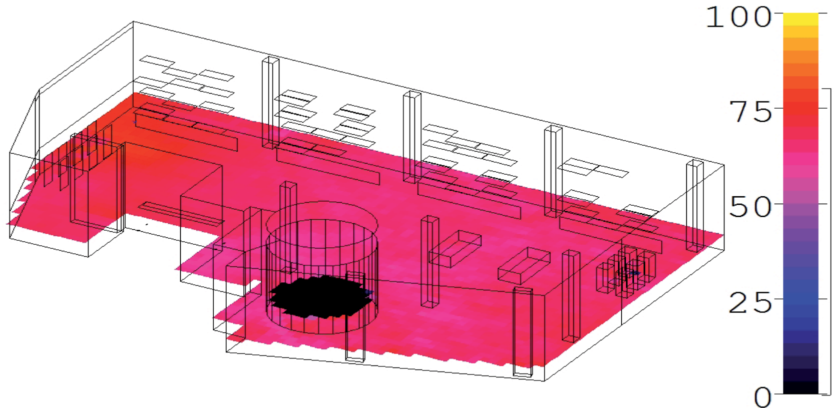
1 RASTI [%]
