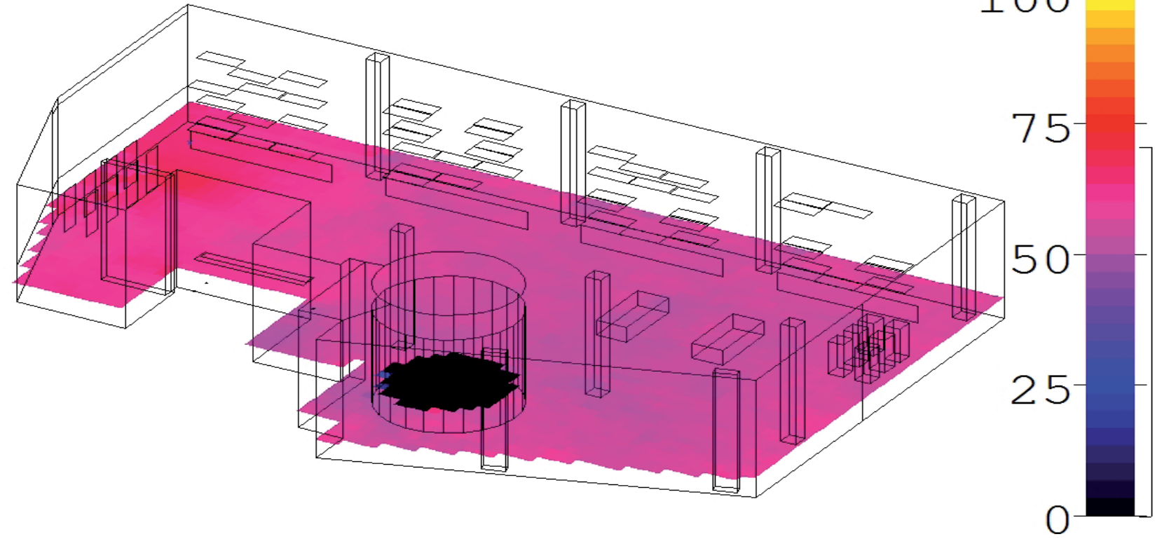
1 RASTI [%]
